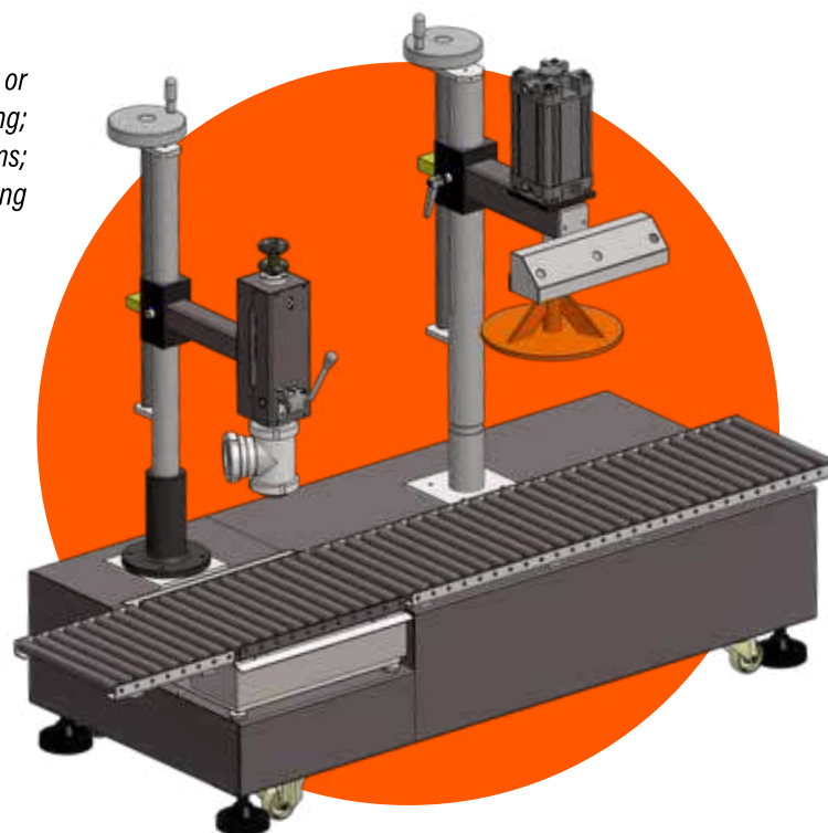
avvitatore screwing machine
